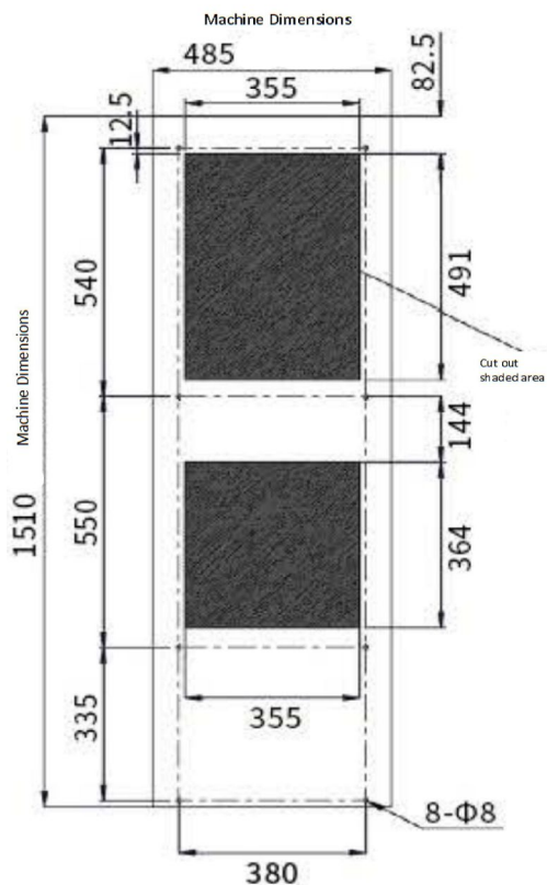
Рис. 1 - Размер для вырезания двери
